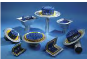
Harmer AV and Harmer Detail Outlets
