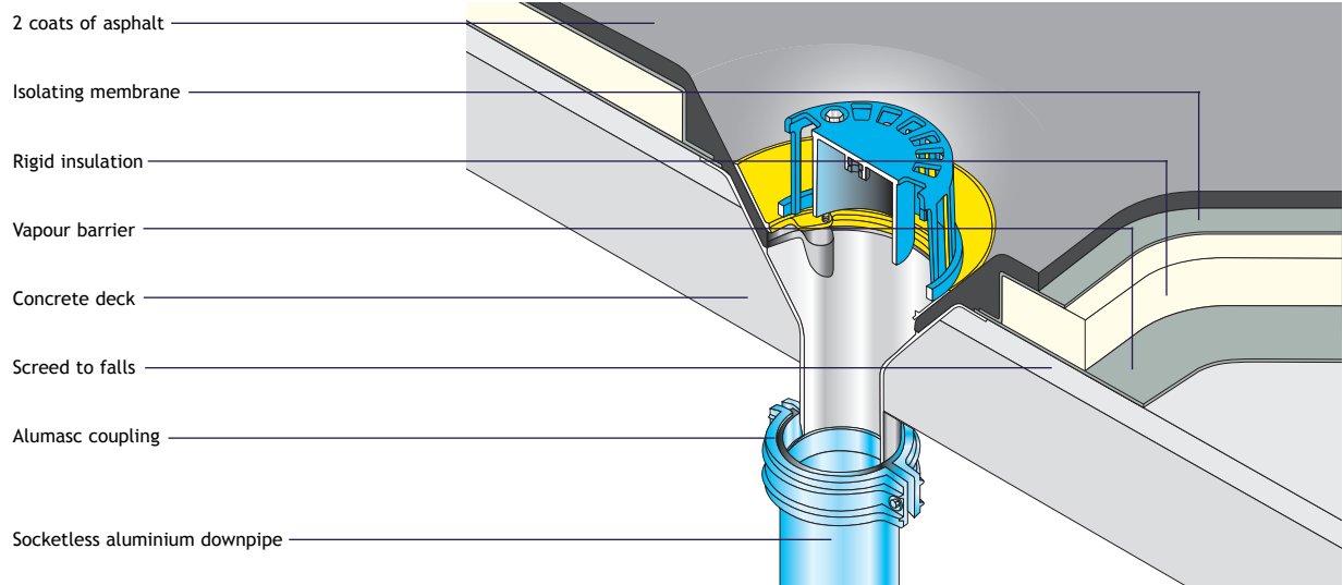
Harmer AV Vertical Spigot Outlet in Warm Roof
