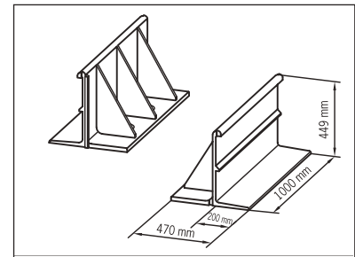
ACO LEP 100
