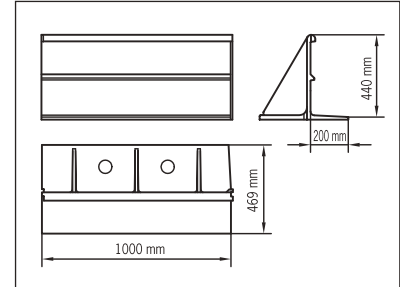
ACO LEP 100
