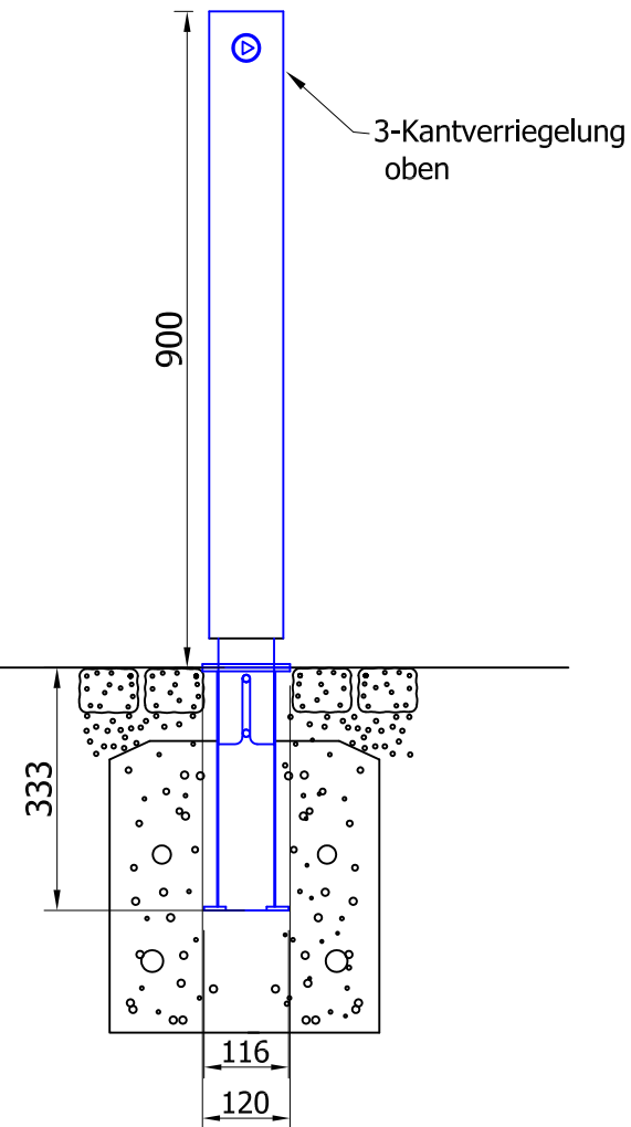
Poller zum Herausnehmen
