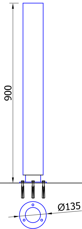
Poller zum Anschrauben
