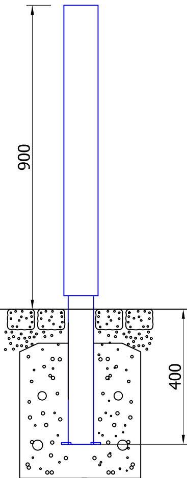
Poller zum Einbetonieren
