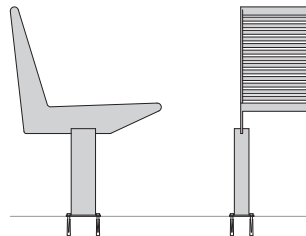
Anschrauben Bolt-on
