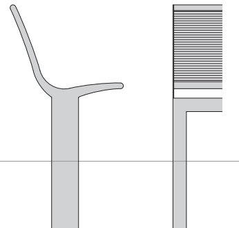
Einbetonieren Concrete-in
