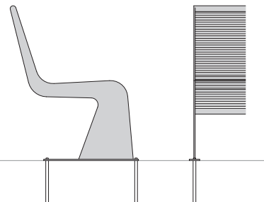
Einbetonieren Concrete-in
