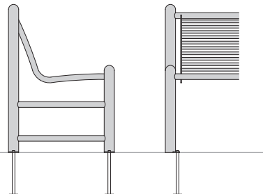
Einbetonieren Concrete-in
