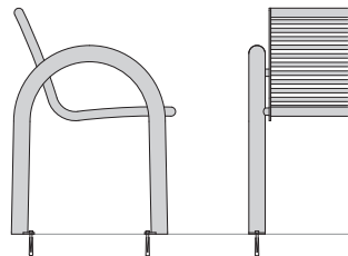
Anschrauben Bolt-on
