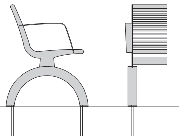
Einbetonieren Concrete-in
