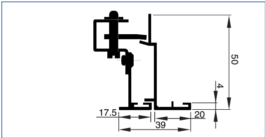
Front border RC-AE-...-0
