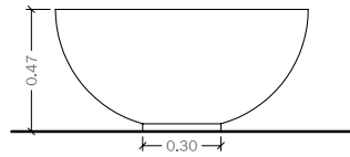
Alçat
