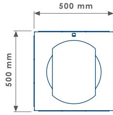
DOME TOP (DT) LOCKABLE
